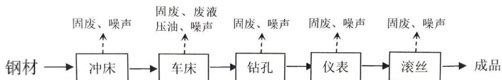
图 2-4 生产工艺流程及产污环节图
