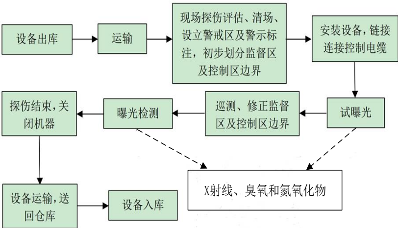
图 9-3 探伤工艺流程及产污环节示意图
