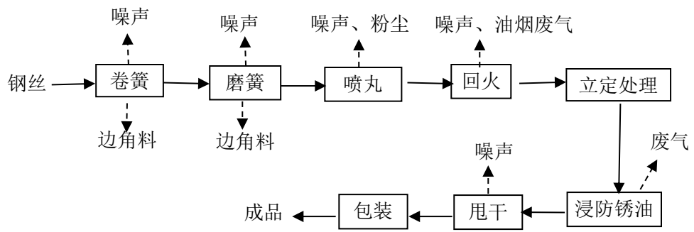
图 2-1 弹簧生产工艺流程图
