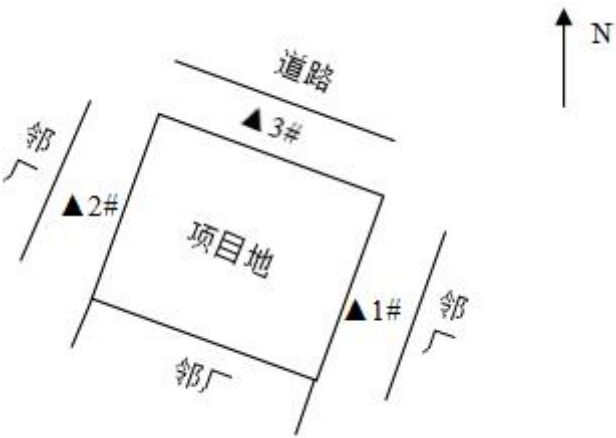
图 7-1 噪声监测点位布置图
