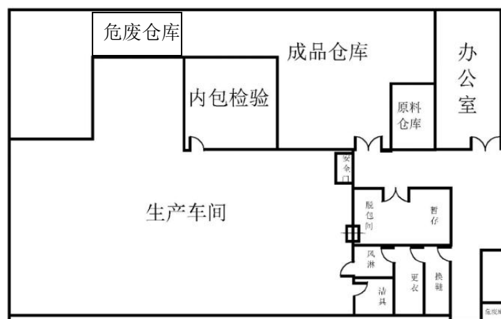
图 3-2 平面布置图
