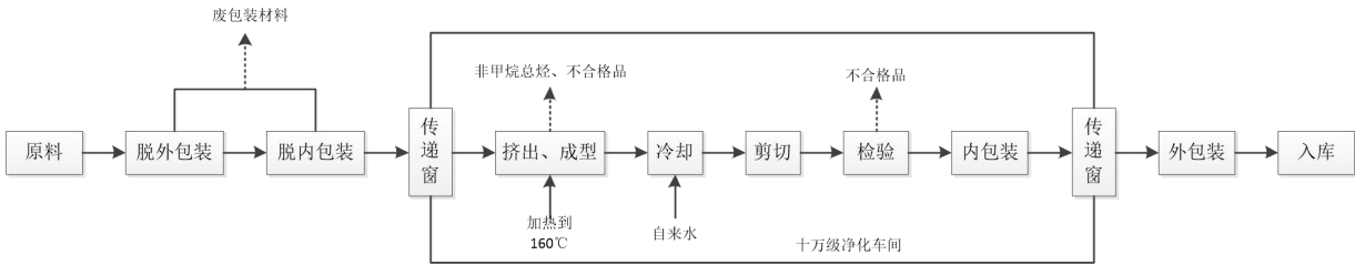
图 3-4 生产工艺流程图
